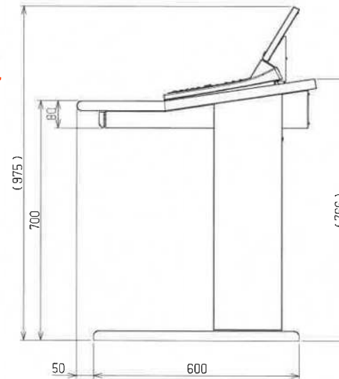
卓上型局線中継台
