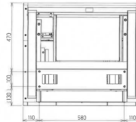
正面
