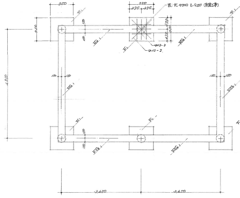
基 礎 伏 七 圖 8:1:50
