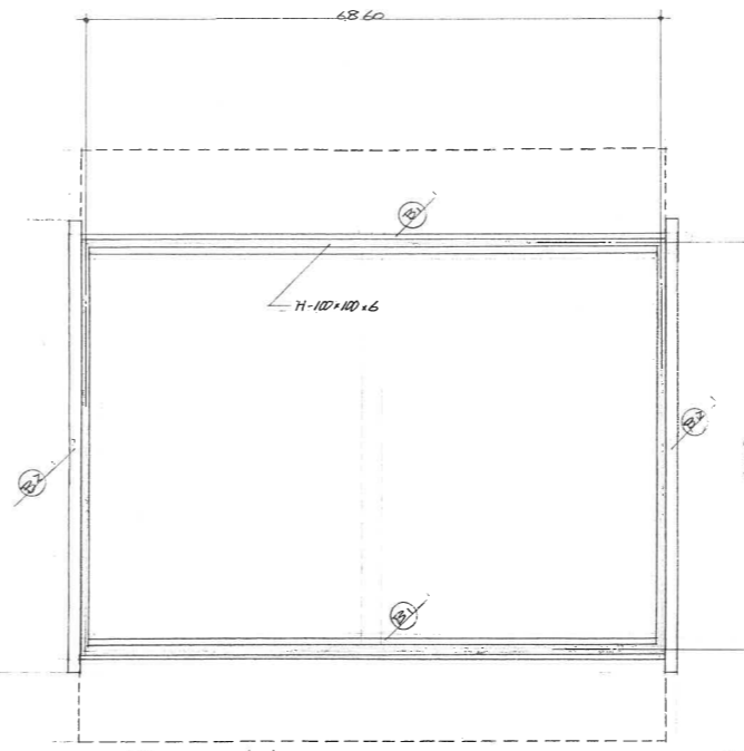
小 屋 伏 七 圖 8:1:50
