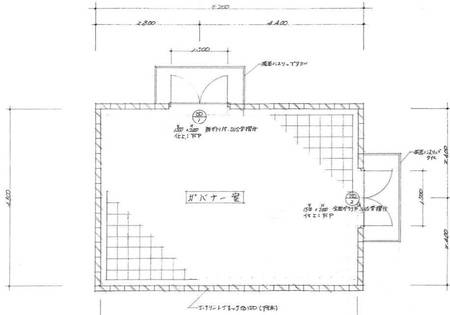
平面図 8:1:50
